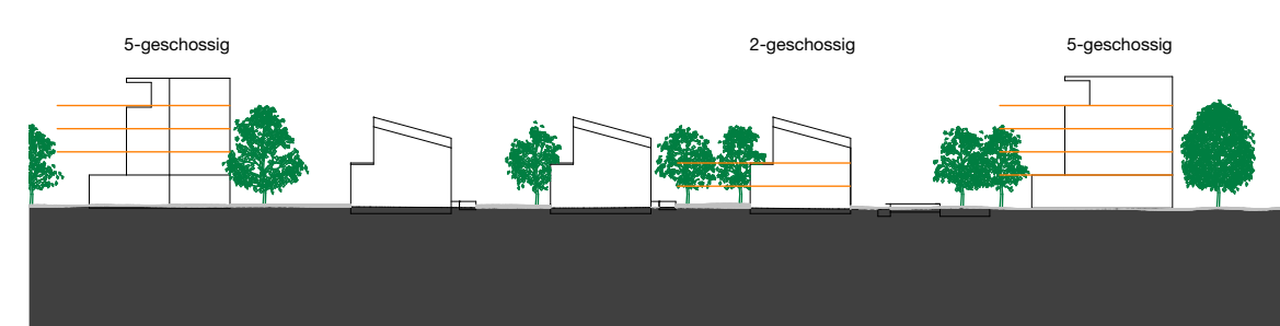
Schnitt 6-6
